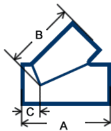
45° lateral
